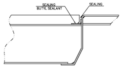
GOOSENECK 1:4
